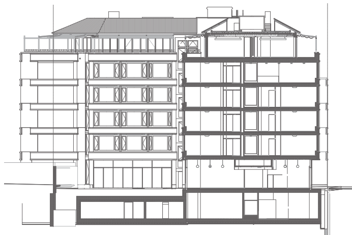
Schnitt
